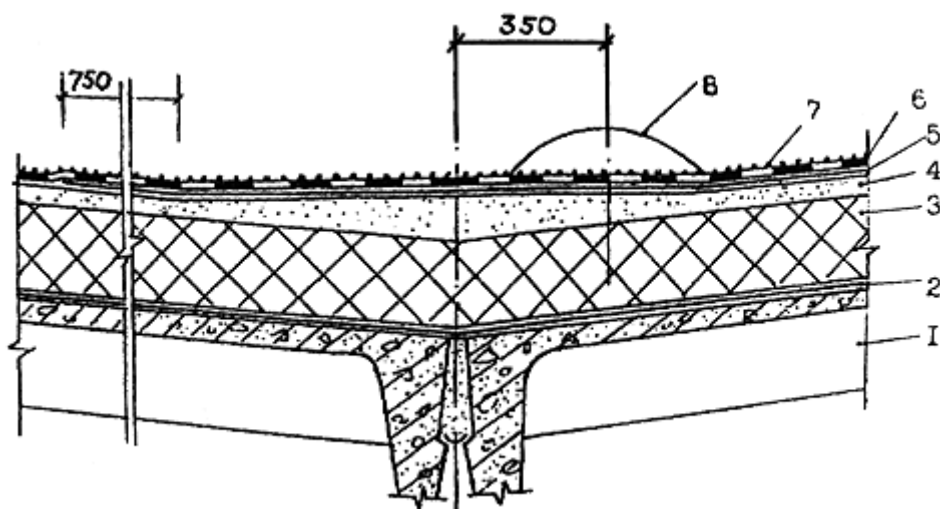
Рис. 8. Ендова кровли
