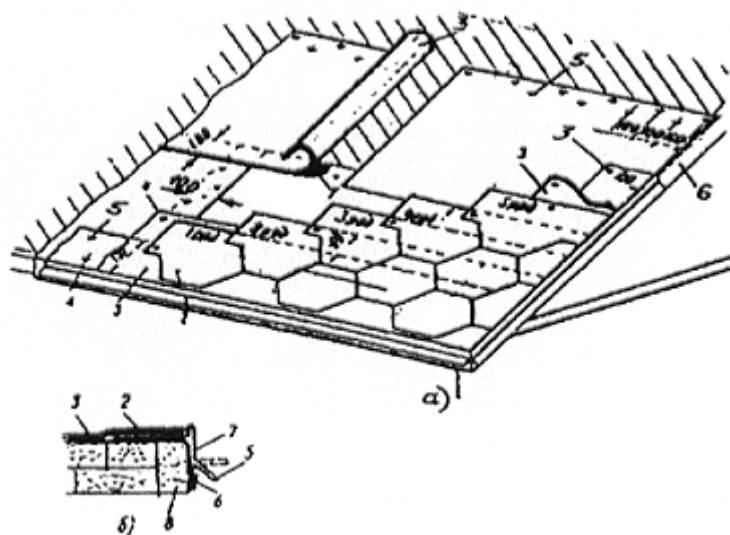
Рис. 20. Конструктивное решение кровли из битумных плиток (шинглы)
