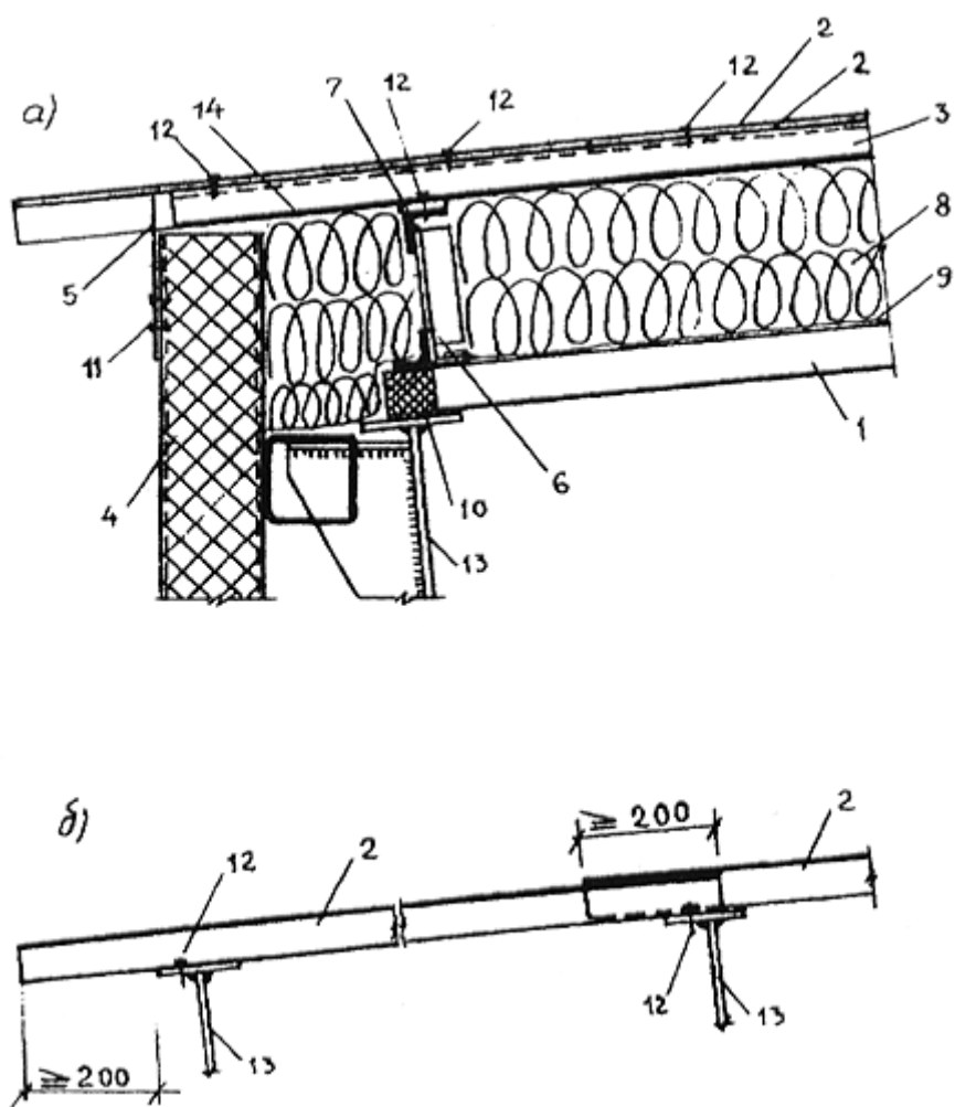
Рис. 26. Карниз кровли из металлического профнастила
