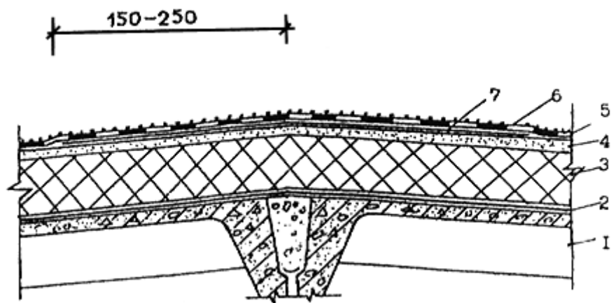
Рис. 7. Конек кровли
