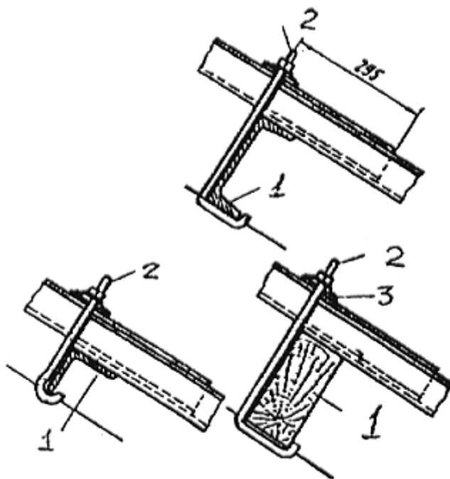
Рис. 15. Способы крепления асбестоцементных волнистых листов к прогонам
